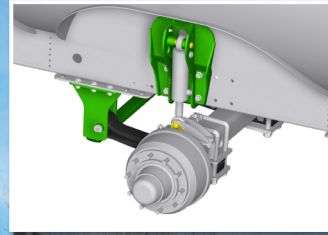
Hydro-Tandem: hydraulische vering van de assen
