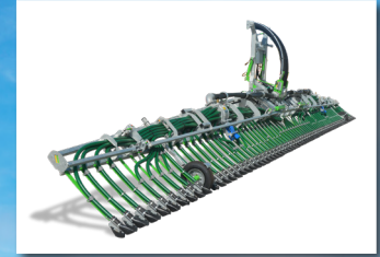
PENDSLIDE PRO 150/60PS2 verspreidingsboom van 15 m
